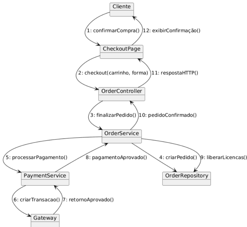
Diagrama de Comunicação - Finalizar Pedido
