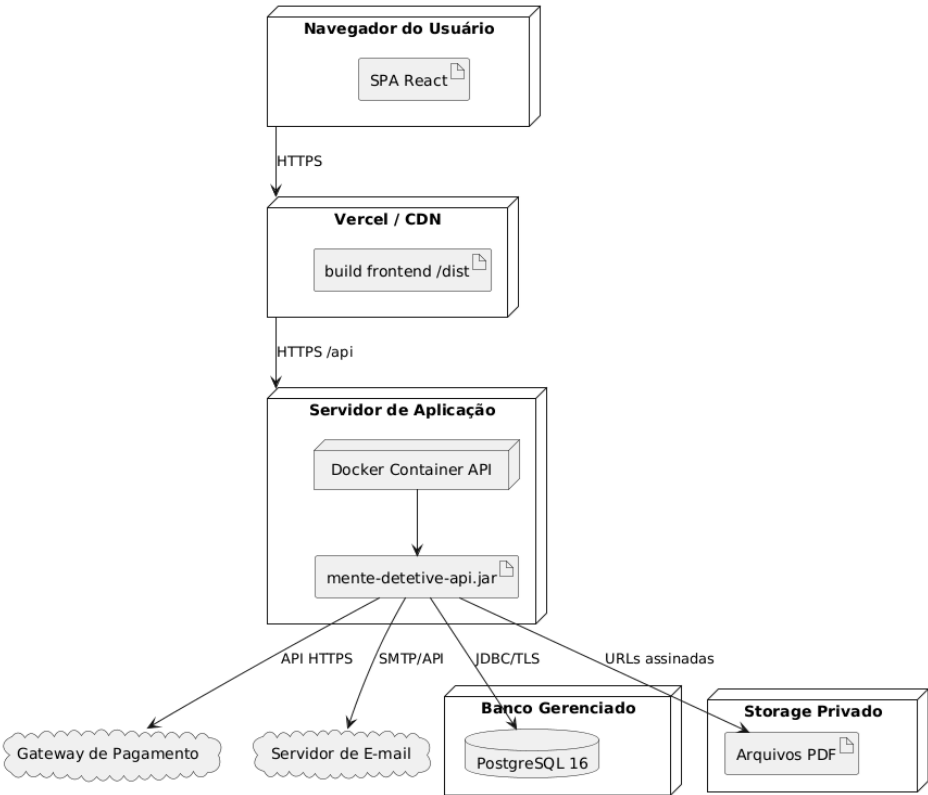
Mente Detetive - Diagrama de Implantação
