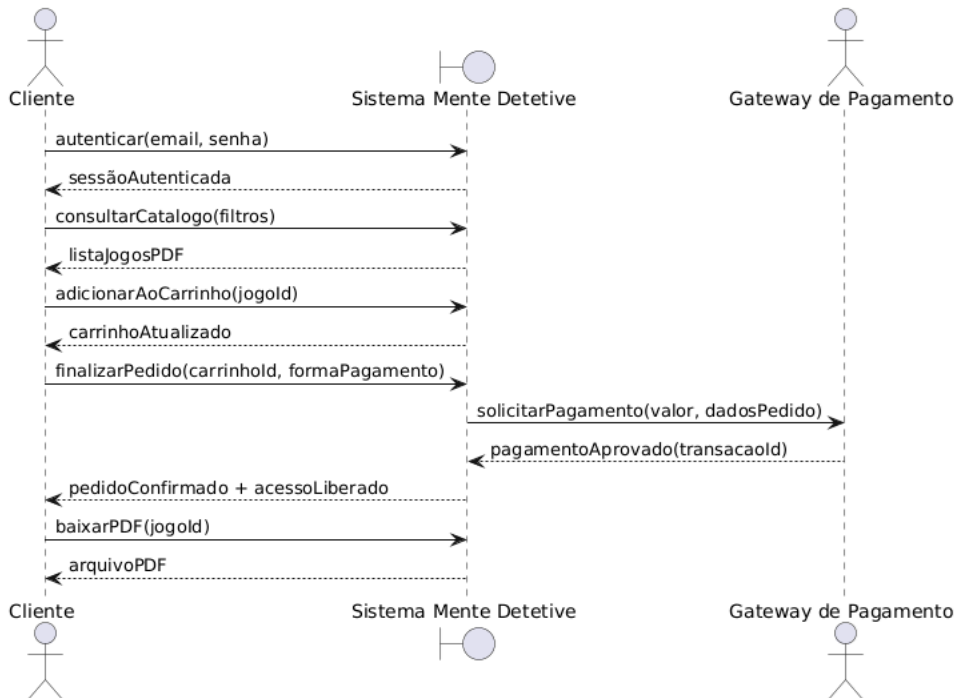
SSD - UC-06 Finalizar Pedido e Comprar PDF
