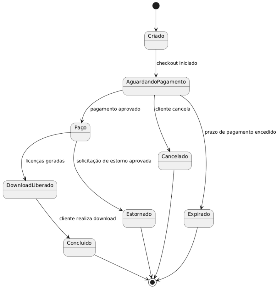
Diagrama de Estados - Pedido
