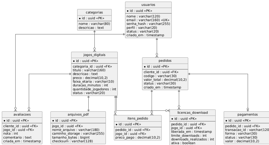
Mente Detetive - Modelo de Dados / DER
